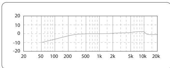
Pasma przenoszenia
